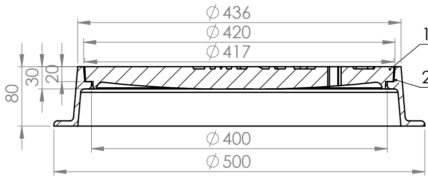
PRZEKRÓJ A-A SKALA 1 : 5
