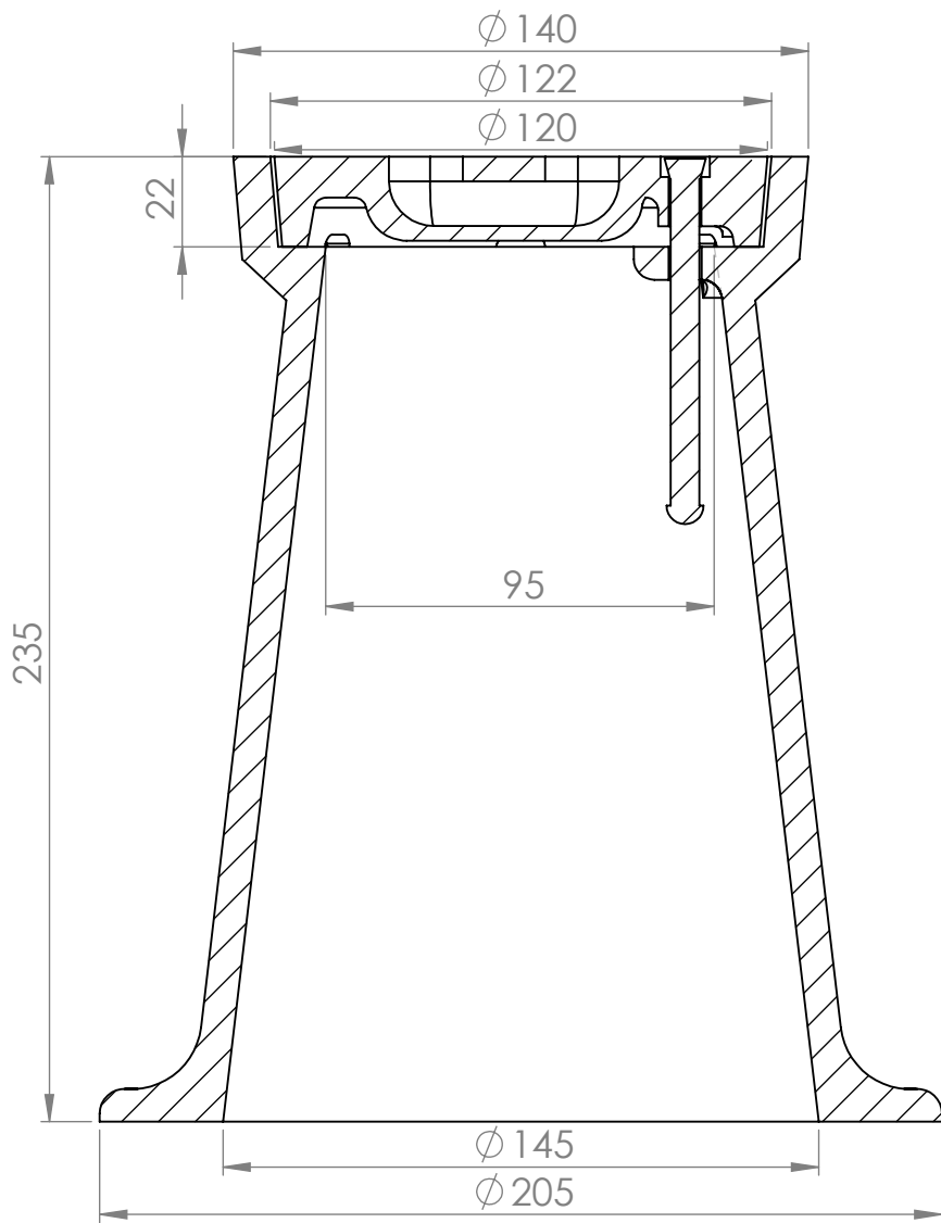
PRZEKRÓJ A-A SKALA 1 : 2
