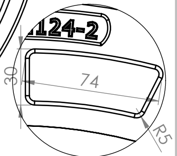
SZCZEGÓŁ A SKALA 1 : 2
